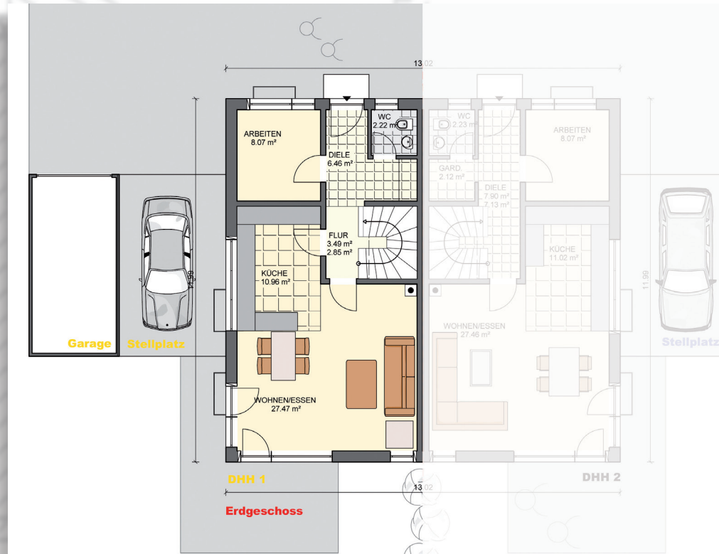
Erdgeschoss
