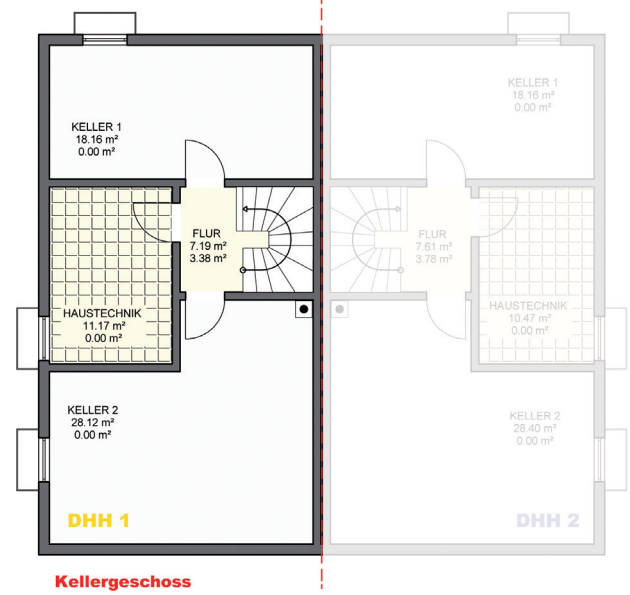
Kellergeschoss
